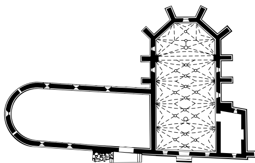
ŚWIDNICA. RZUT KOŚC. ŚW. BARBARY (OB. KLUB NOT) wg: Hanulanka...
