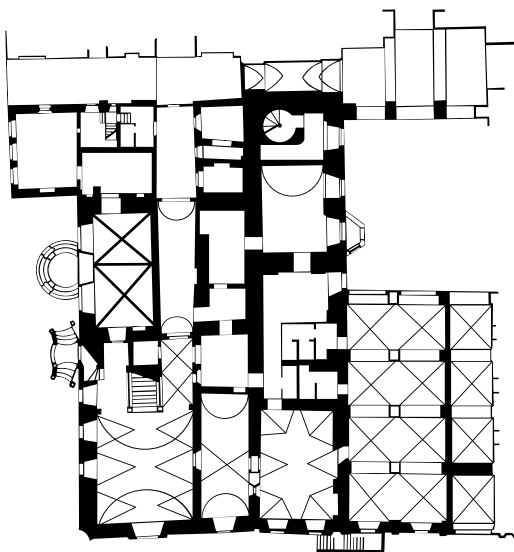
ŚWIDNICA. RZUT RATUSZA wg: Pilch, Ratusze...
